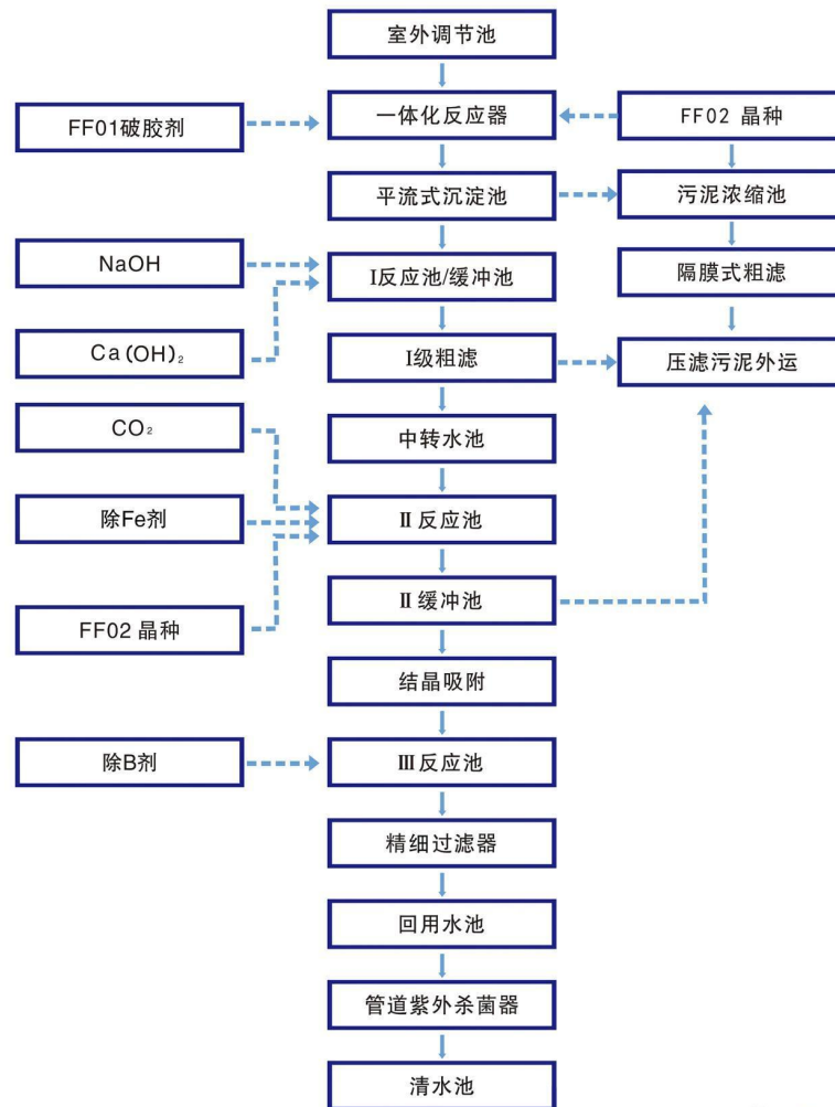
图5-4 水处理工艺流程图
