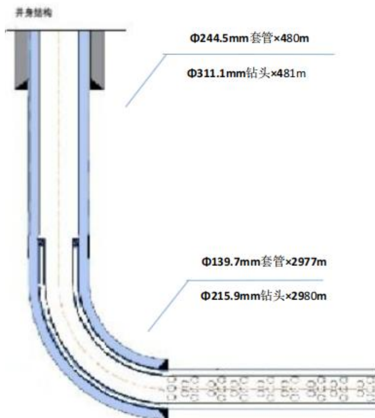
图2-1 水平井井身结构图
