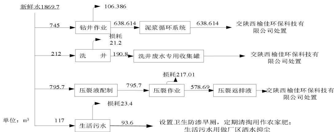
图 2-2 项目水平衡图
