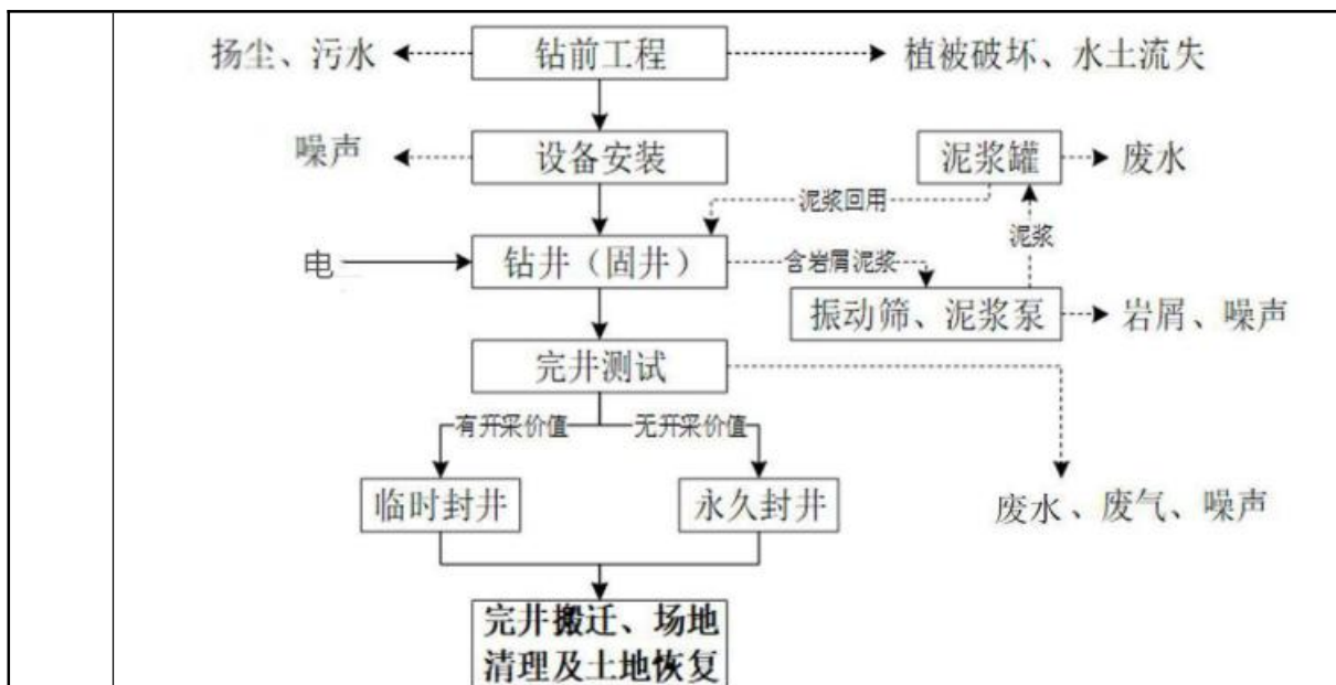
图 2-3 项目主要工艺流程及产污环节图
