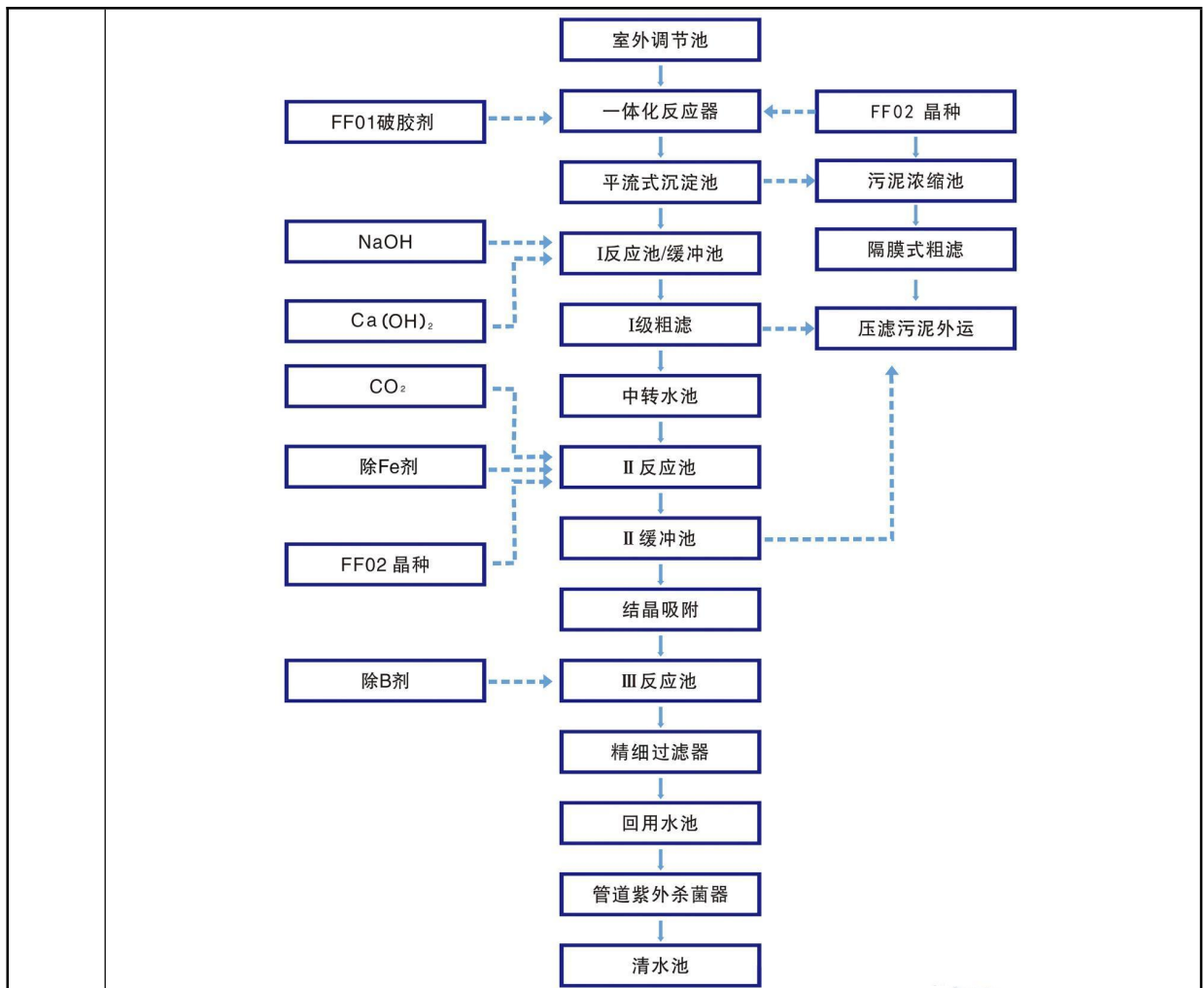
图 5-5 水处理工艺流程图
