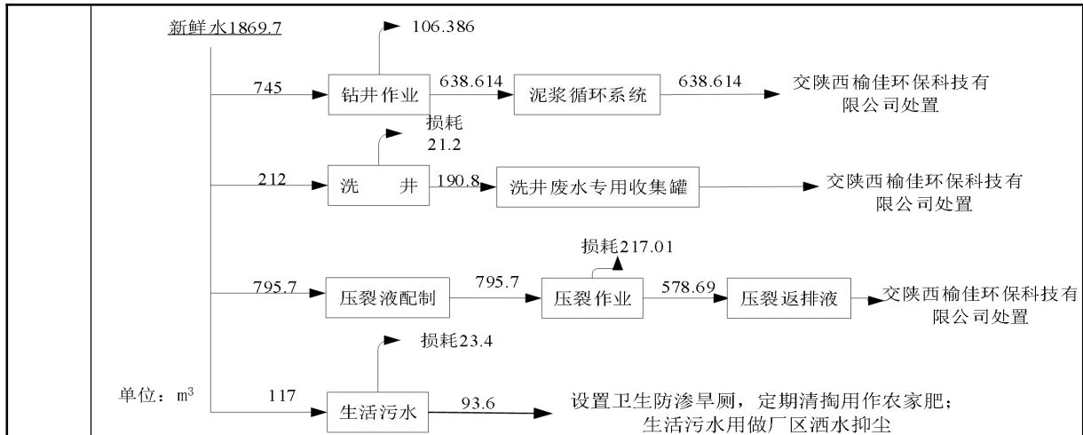
图 2-2 项目水平衡图
