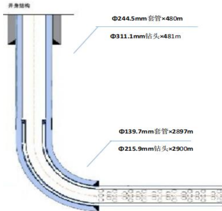
图2-1 水平井井身结构图
