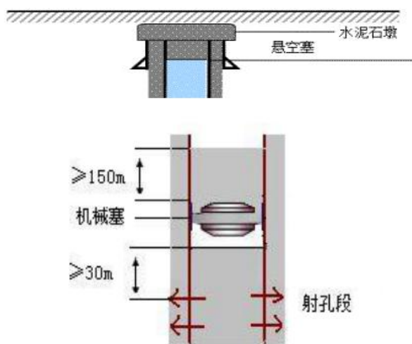
图 2-4 井口及射孔封堵示意图
