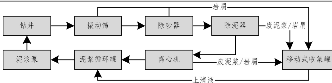
图 2-3 泥浆闭路循环系统示意图
