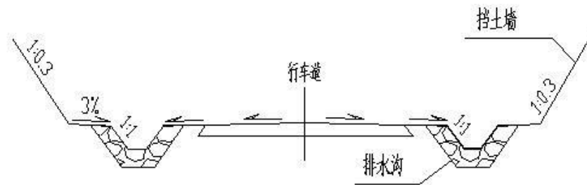
图 5-5 路堑边坡防护示意图
