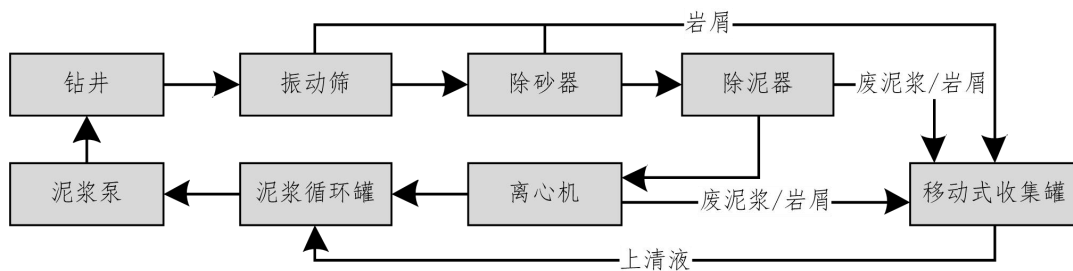
图 2-4 泥浆闭路循环系统示意图
