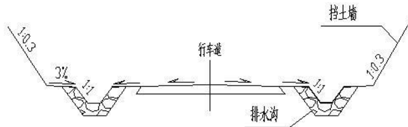
图 5-4 路堑边坡防护示意图
