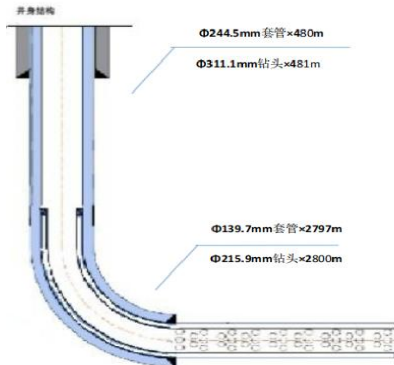
图2-1 水平井井身结构图
