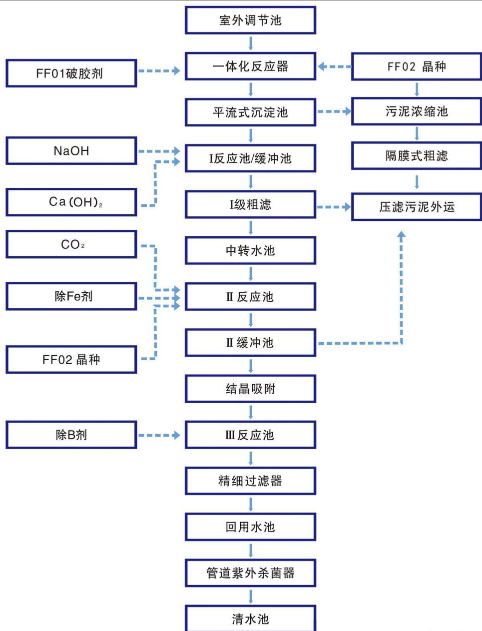
图 5-3 水处理工艺流程图
