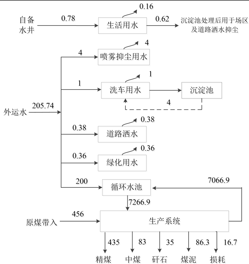
图 1 项目水平衡图
