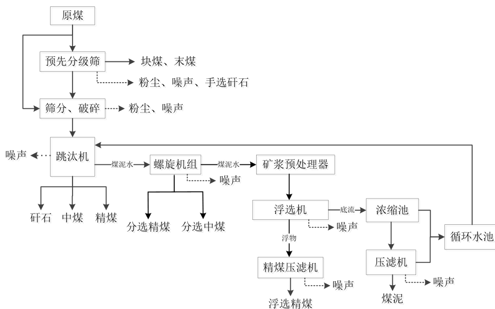
图 3 80 万吨/年洗选生产线工艺流程及产污节点图
