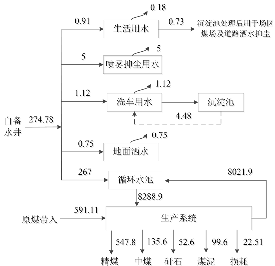
图 1 项目水平衡图
