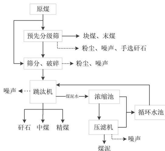
图 2 40 万吨/年洗选生产线工艺流程及产污节点图
