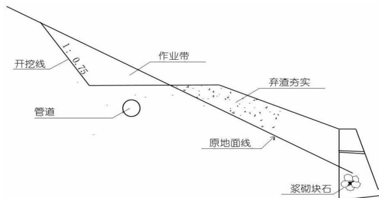
图 8 管道横向敷设图
