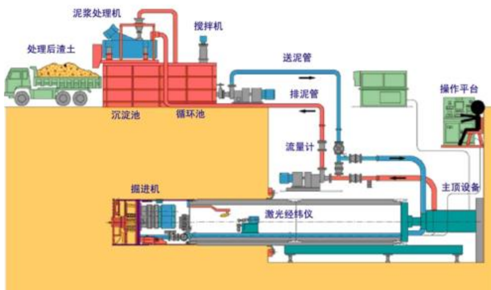
图6 顶管施工断面示意图
