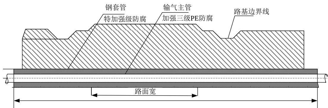
图 7 沥青路穿越施工方式断面示意图
