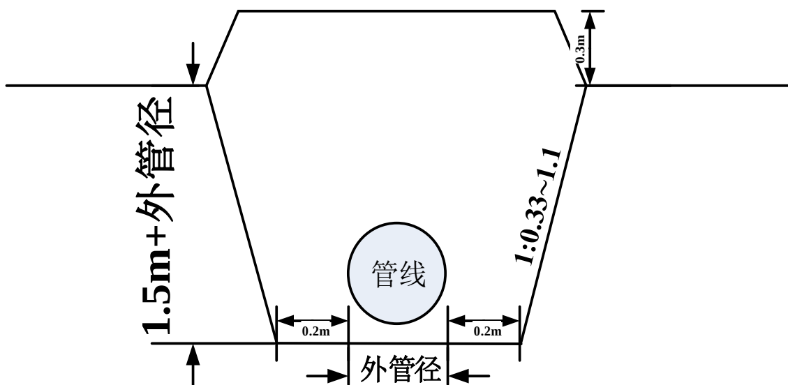
图5 管沟横断面示意图
