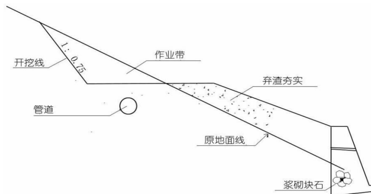
图 9 管道横向敷设图
