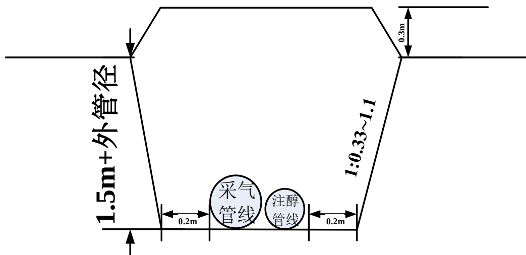
图 4 单管管沟横断面示意图
