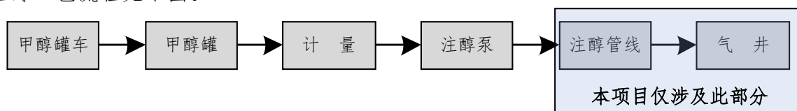
图 5 注醇工艺流程示意图
