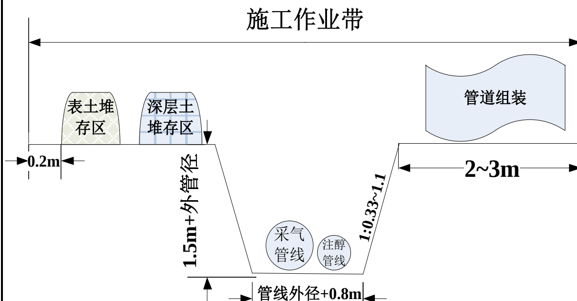
图 3 单管施工作业带断面示意图
