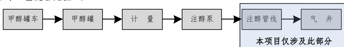
图 7 注醇工艺流程示意图
