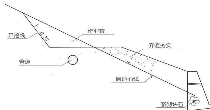
图9 管道横向敷设图
