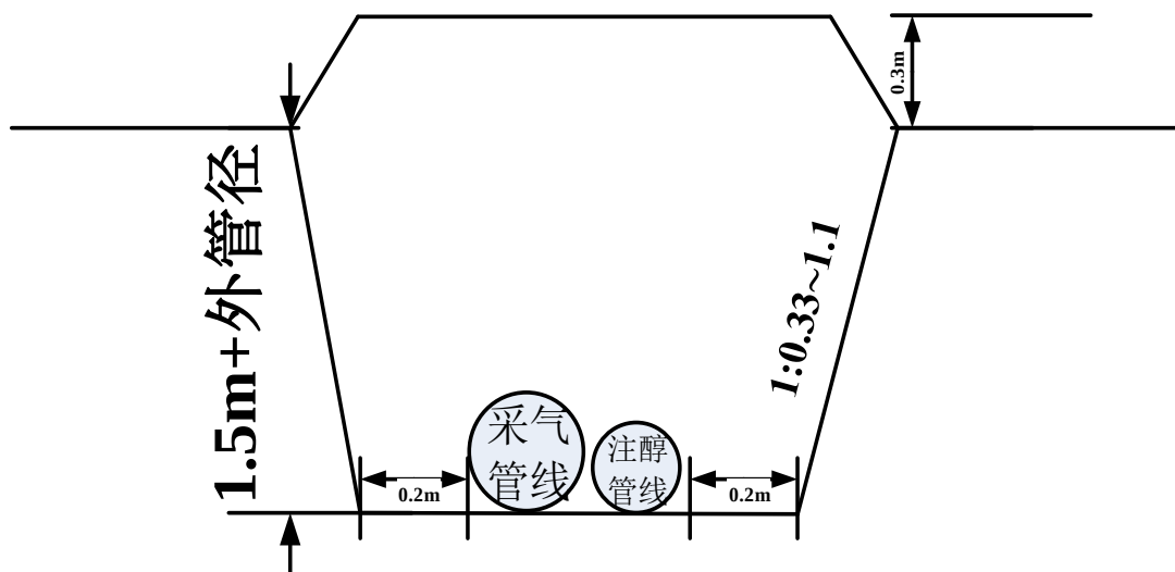
图 4 管沟横断面示意图
